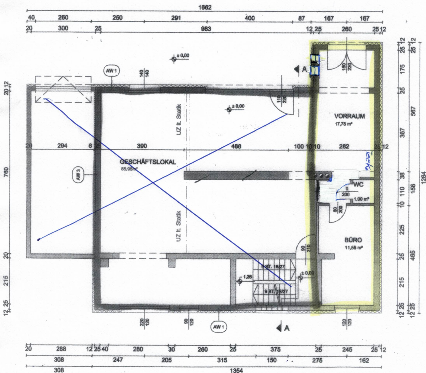
GRUNDRISS ERDGESCHOSS
